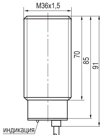
Габаритный чертёж
